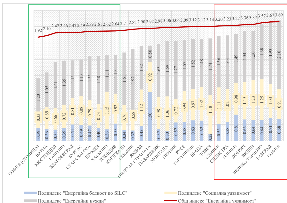
Фигура 8: Общ индекс „Енергийна уязвимост на домакинствата в България“ по области, 2023 г.
